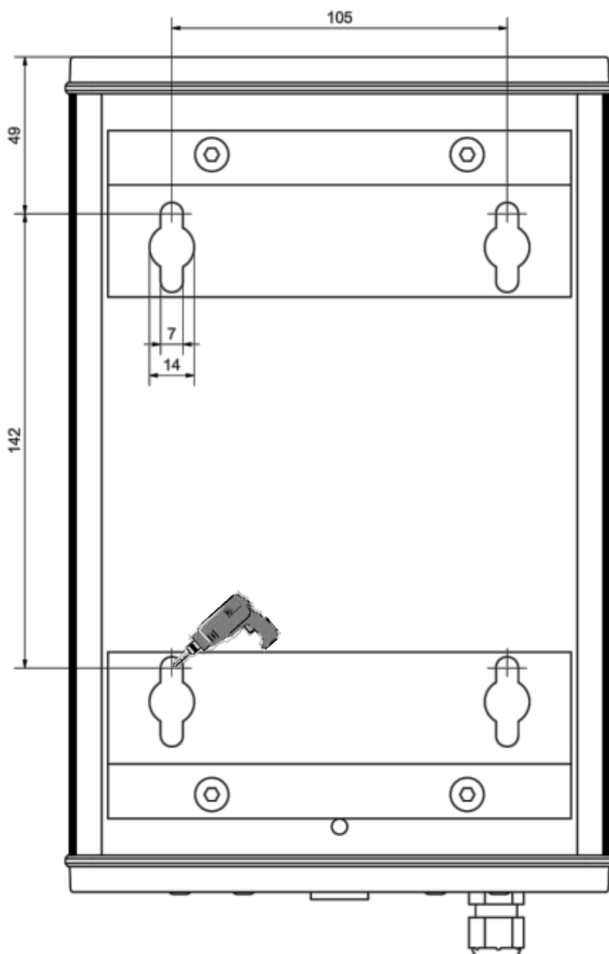
Borrschablon ALF® - Tronik vägg enhet (Denna ritning är ej skalendig)
